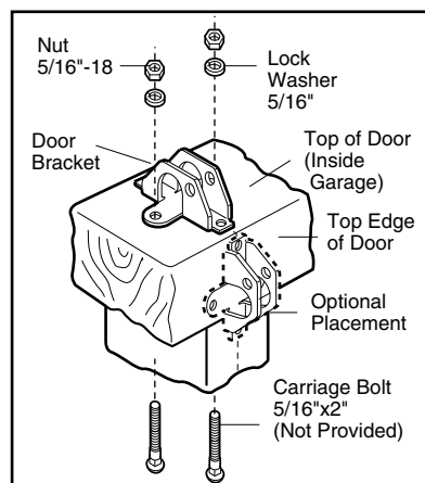
WOOD DOOR
